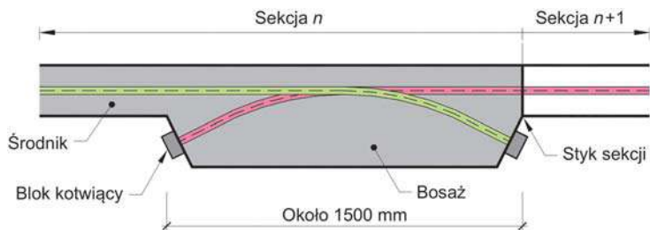
Rysunek 3.32. Przekrój poziomy środnika w miejscu łączenia kabli wypłutu na zakład
