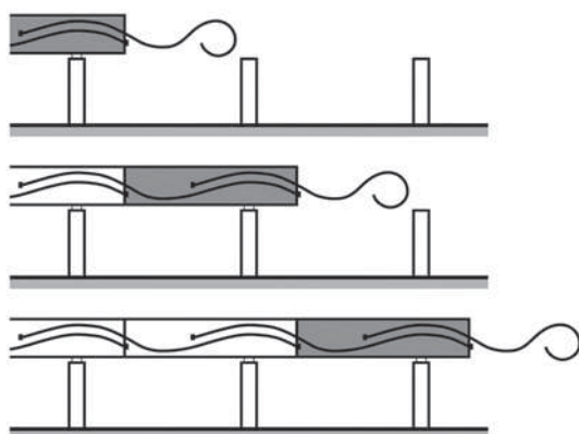
b) Kable prowadzone przez dwa segmenty
