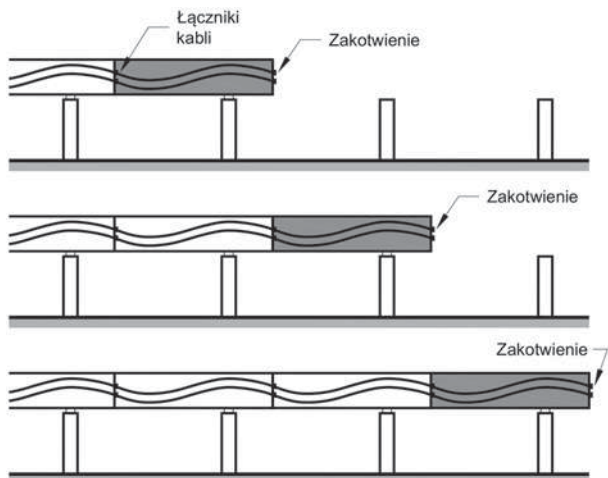
a) Kable prowadzone na odcinku jednego segmentu (kotwienie wszystkich kablów na czole wykonanego segmentu)
