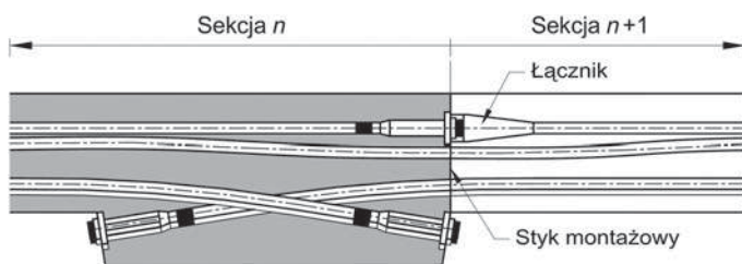
Rysunek 3.34. Mieszany układ kabli w styku segmentów
