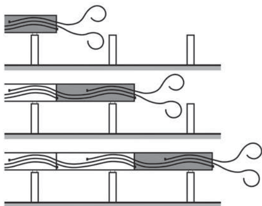
c) Kable prowadzone przez trzy segmenty
